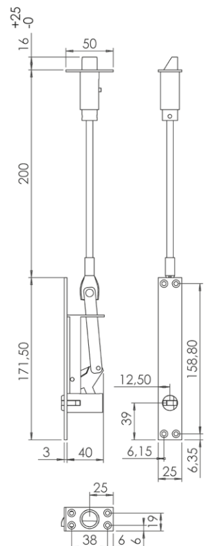
Måttskiss STEP 22.
