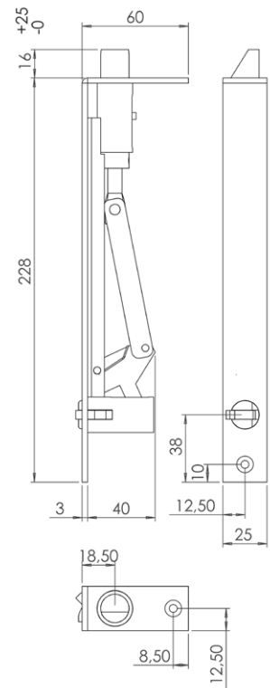
Måttskiss STEP 21.
